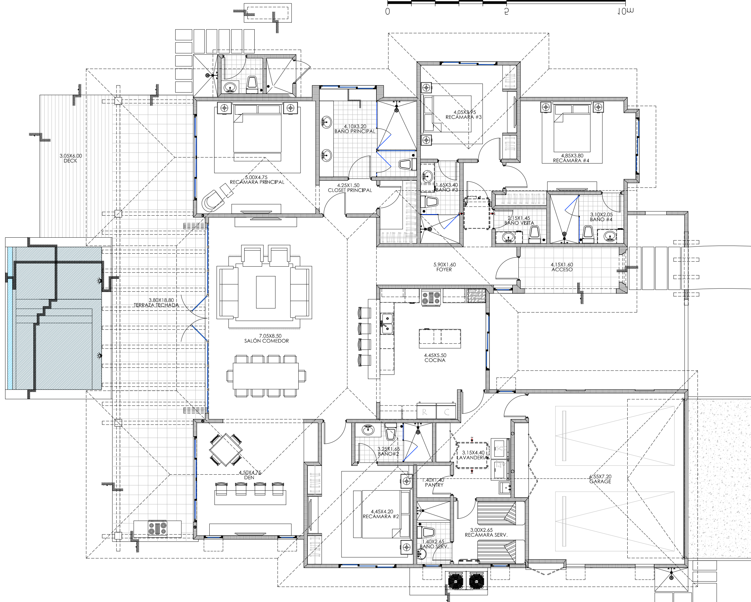
PLANTA ARQUITECTÓNICA
